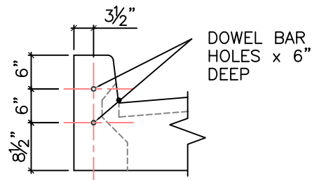
END ELEVATION
