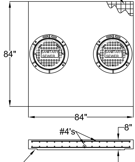
CONVERSION LID
